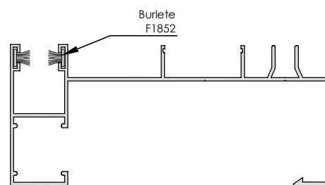
Cerco lateral int. + guía (testa) 6551
