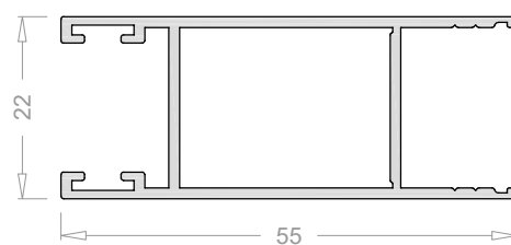
Hoja lateral 19 mm 6509
