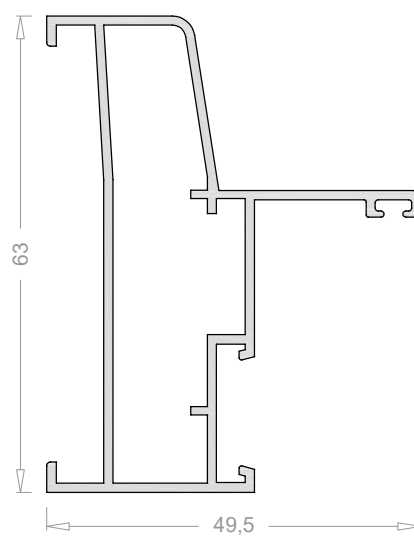
Cerco para fijo perimetral 6569
