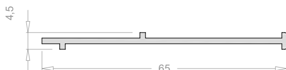
Perfil unión cercos (6500+3500) 6515
