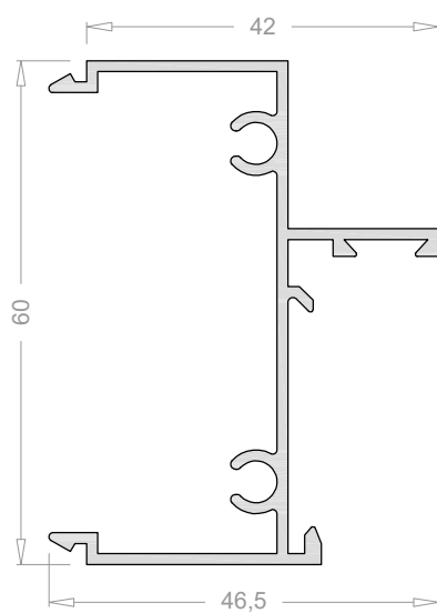
Cerco para fijo (junquillo 3500) 5361
