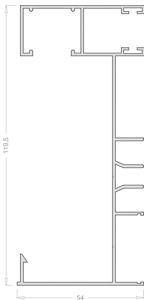
Cerco lateral ext. con guía a testa 6550
