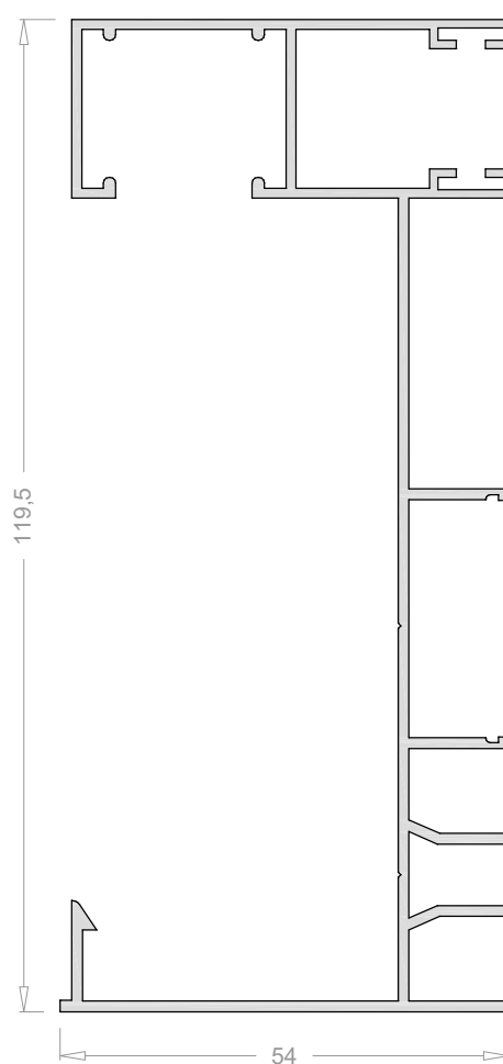
Cerco lateral int. con guía a testa 6551
