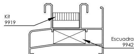
Cerco perimetral 6567
