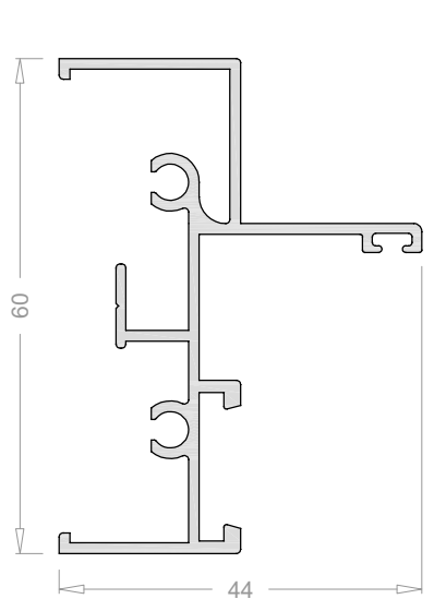
Cerco para fijo con portatornillos 6524
