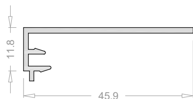
Vierteaguas superior 6805
