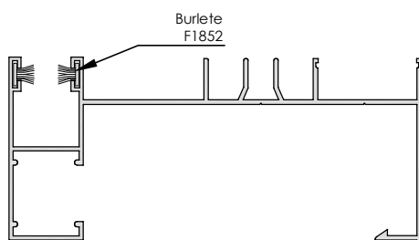
Cerco lateral ext. + guía (testa) 6550
