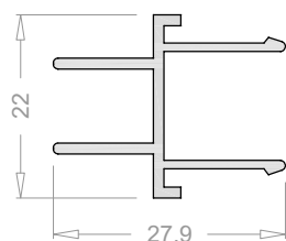
Acople hojas enfrentadas 6516
