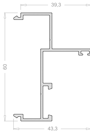
Cerco para fijo 6525
