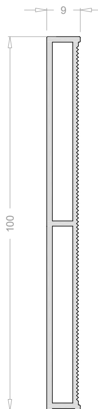
1357 Rodapie de 100 mm
