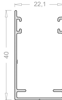
Guía mosquitera 40 mm 2428 Pedido mínimo 840 mts
