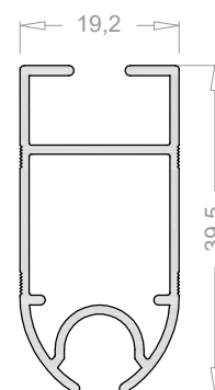
Palillo para toldo 2493 Pedido mínimo 630 mts
