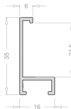
Moldura 35 mm 2443
