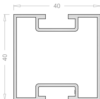
Perfil 40x40 con 2 calles opuestas 2472
