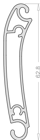
Lama de 63 mm 2424
