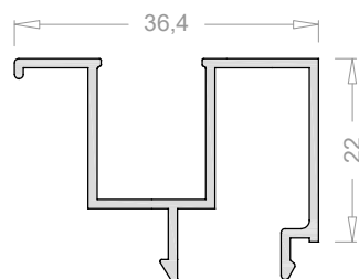
Bastidor para lamas (S2500) 2422
