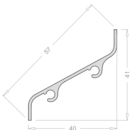
Lama con portatornillos 2456
