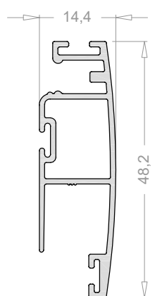
Mosquitera curva 2497
