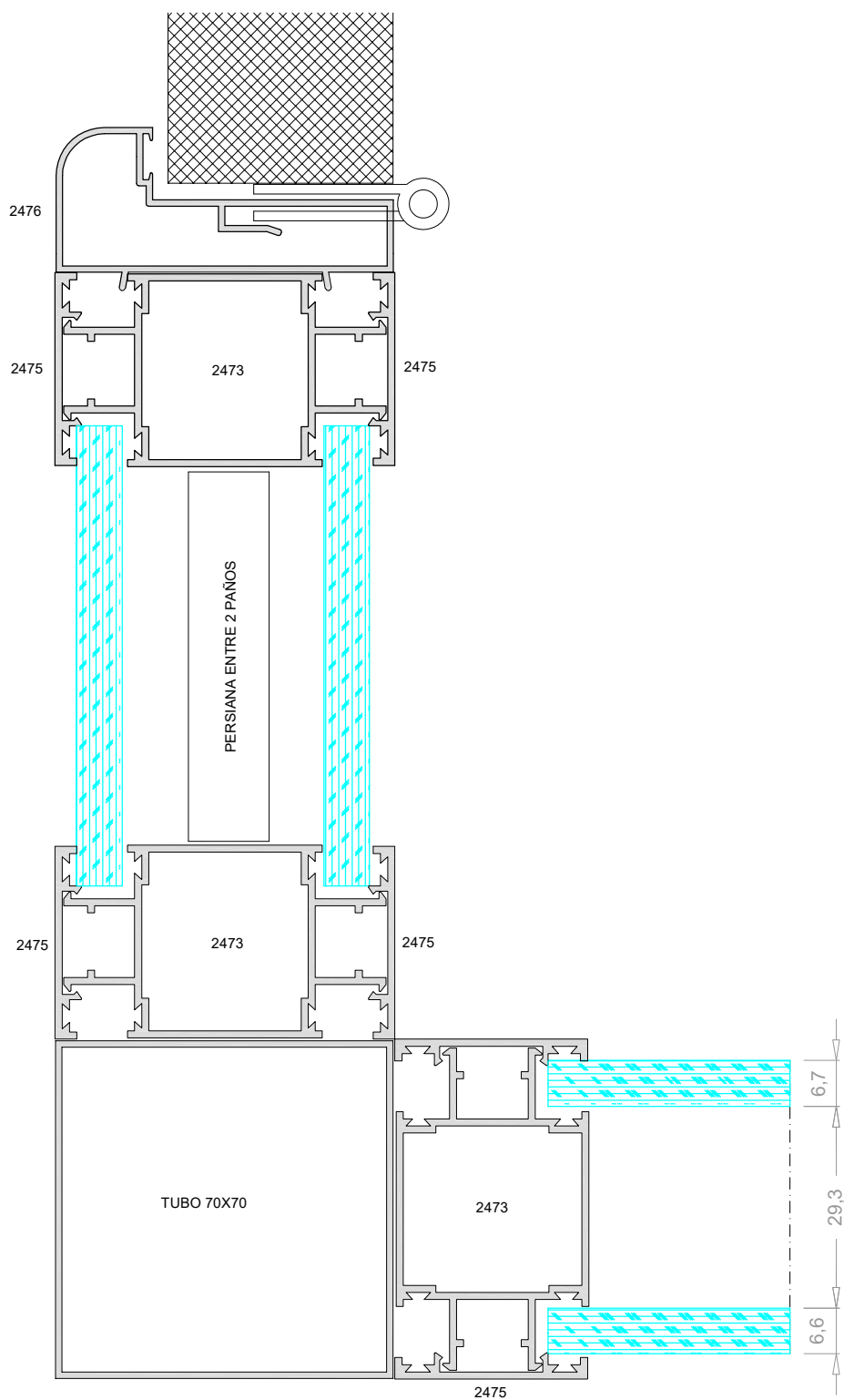
División de oficina doble
