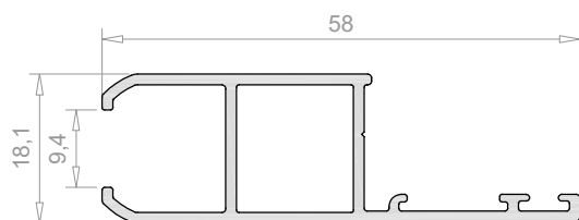
Hoja para frailer 2465
