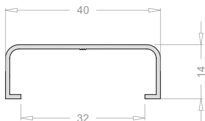
Perfil Tapa 2484
