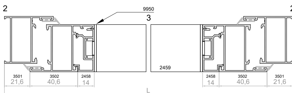
Lama fija. Serie 3500
