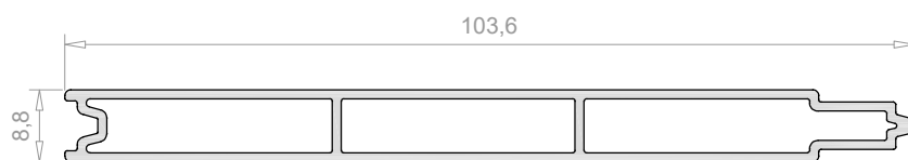
Lama para frailer 2464
