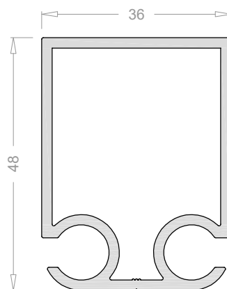
Palillo doble 2455 Pedido mínimo 252 mts
