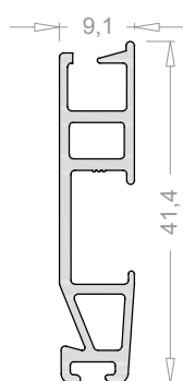
Terminal para mosquitera 2408 Pedido mínimo 750 mts
