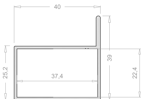
Montante para lamas solapadas 2460
