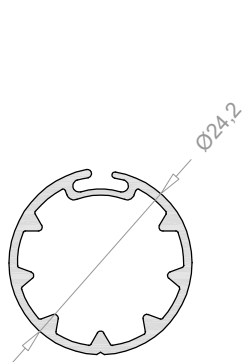
Eje para mosquitera 2407 Pedido mínimo 834 mts
