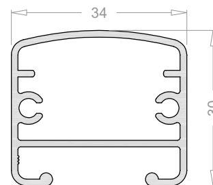
Guía mampara de baño 2415 Pedido mínimo 450 mts
