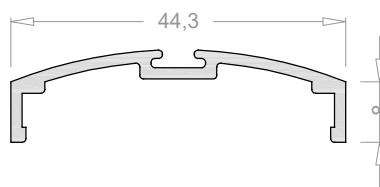
Perfil para puertas vaivén 2451
