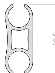
Perfil Intermedio Cortavientos 2308 Pedido mínimo 875 mts
