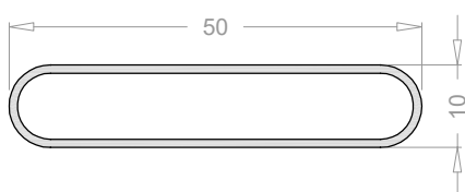
Lama ovalada de 50 mm para celosías 2459
