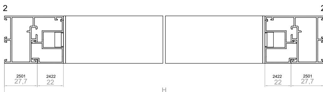
Lama fija. Serie 2500
