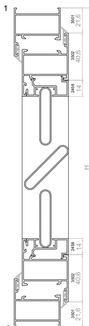
Lama fija. Serie 3500
