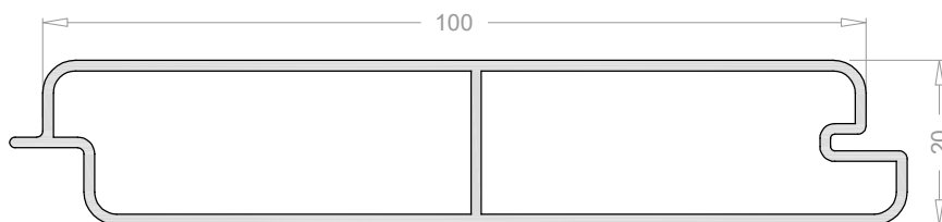
Lama para machihembrar de 100 mm 2462
