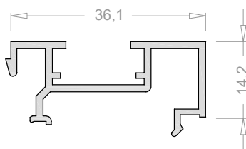
Bastidor para lamas (S3500) 2458
