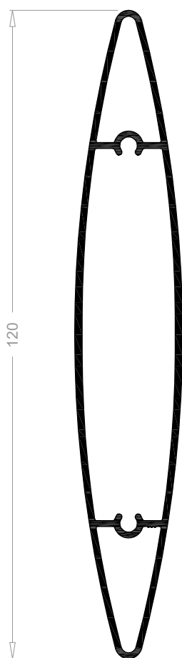
2415 Lama Fija 120 mm Lama de Avión
