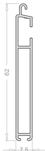
Terminal de 57 mm 2434 Pedido mínimo 696 mts
