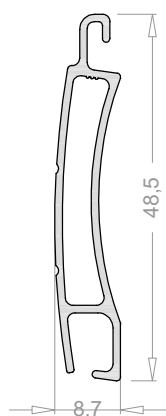
Lama de 42 mm 2467
