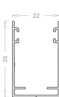
Guía mosquitera 35 mm 2414 Pedido mínimo 930 mts
