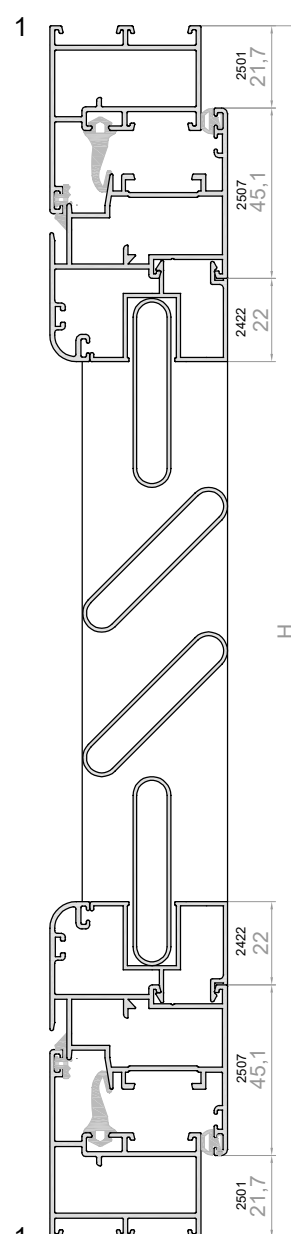
Lama fija. Serie 2500
