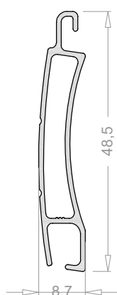
Lama de 42 mm B.E. 2429 Pedido mínimo 936 mts
