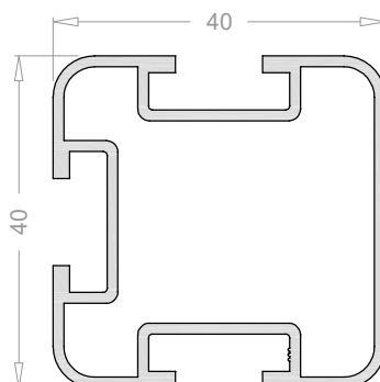
Perfil 40x40 con 3 calles 2495
