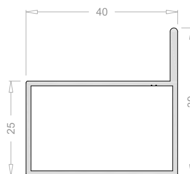
Montante para lamas separadas 2466
