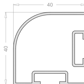
Esquinero redondeado de 40x40 2474
