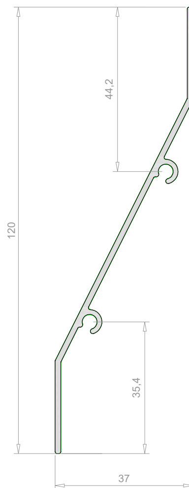
Lama con portatornillos 120 mm 1871
