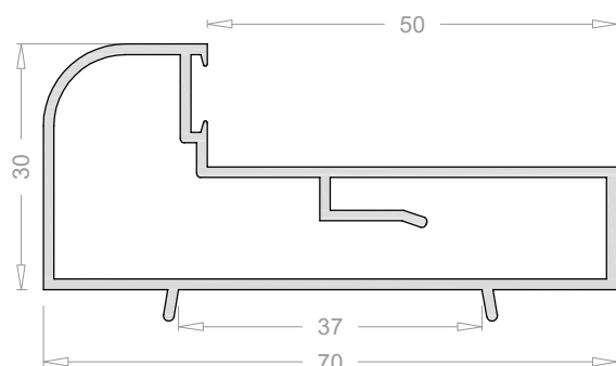
Cerco de puerta 2476
