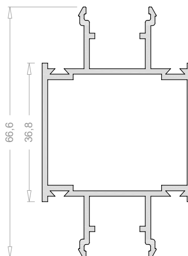
División de oficina (doble acrist.) 2473
