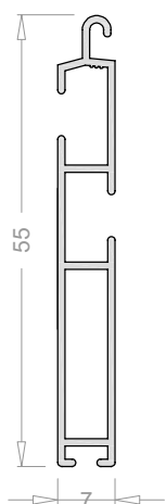
Terminal de 50 mm 2426
