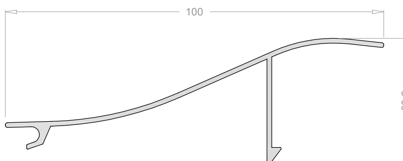
Lama para tendaderos 2461
