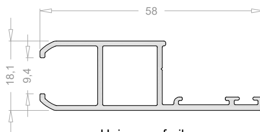
Hoja para frailer 2465
