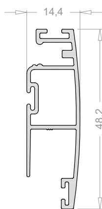
Mosquitera curva 2497
