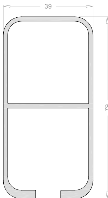
Guía redondeada 80x40 para toldos 2405 Pedido mínimo 186 mts
