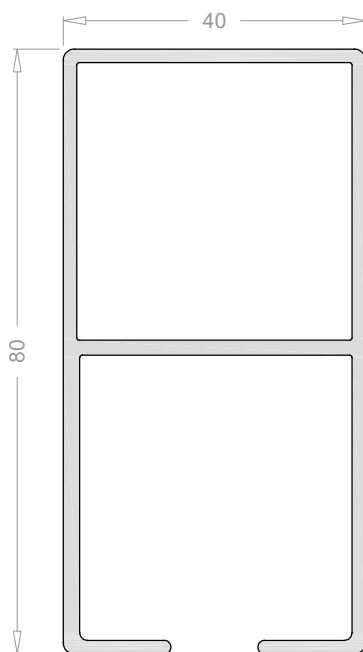
Guía 80x40 para toldos 2454 Pedido mínimo 192 mts
