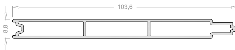
Lama para frailer 2464
