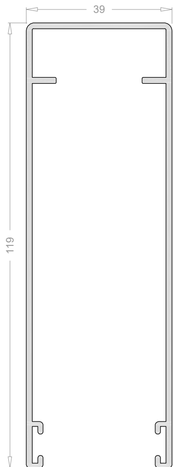
Guía cortavientos de 120 mm 2437 Pedido mínimo 186 mts
