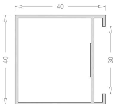
Montante para portalamas 2417
