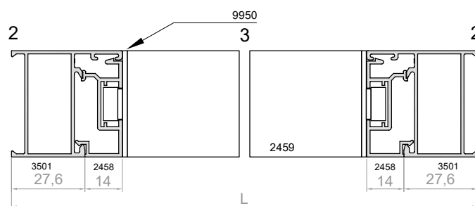
Lama fija. Serie 3500
