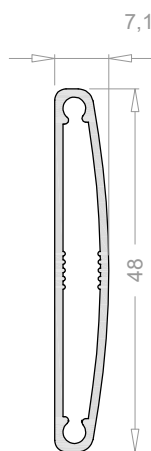
Travesaño 2398
