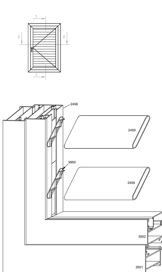
Sistema de lamas para serie 3500
