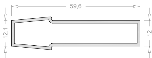
Lama decorativa 2416
