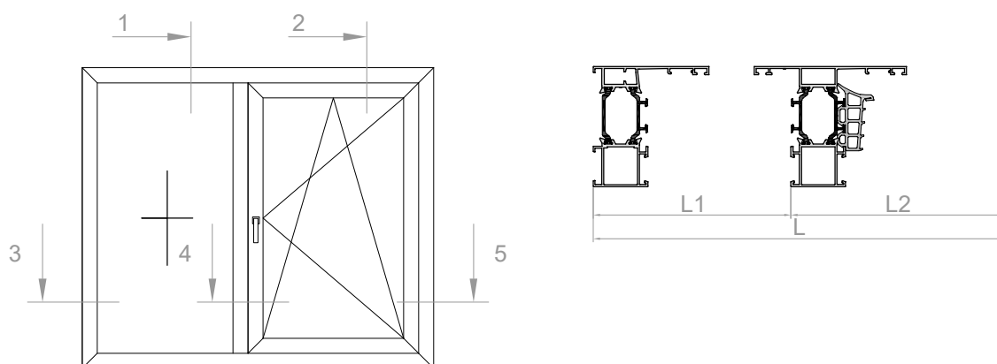
VENTANA - Una hoja + fijo
