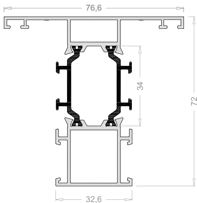
Travesaño de 77 mm 4307
