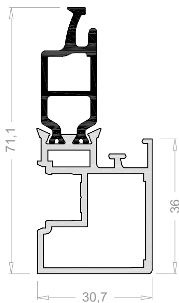
Hoja Inversora 31 mm 3303
