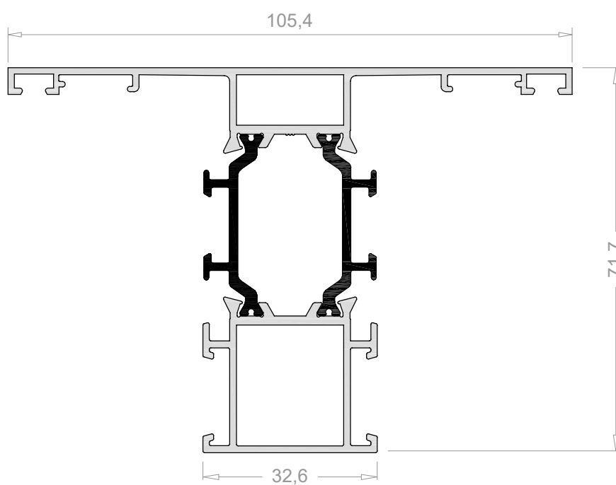
Travesaño simétrico de 105 mm
