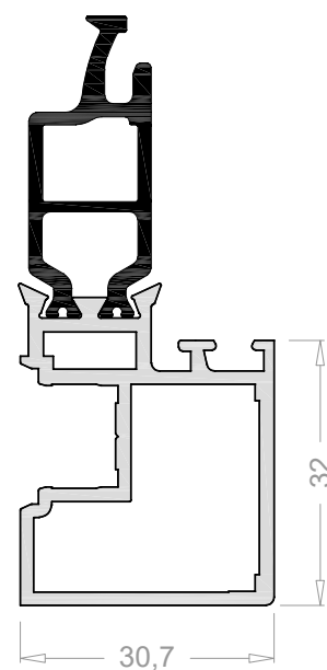
Hoja Inversora 35 mm 3305
