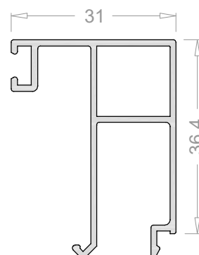
Junquillo recto alto de 31 mm 3313
