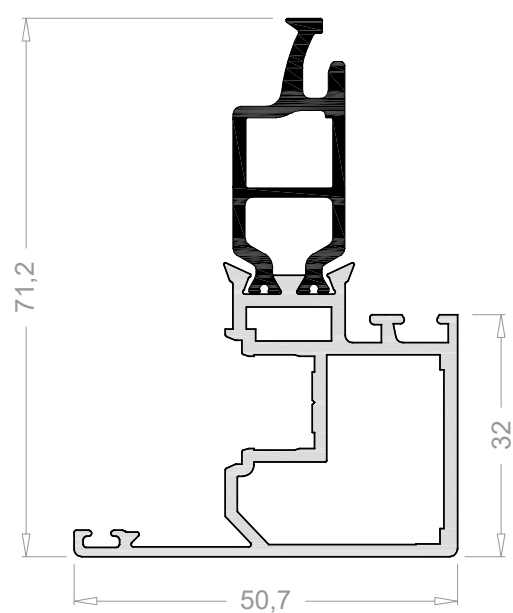
Hoja Recta 35 mm 3304
