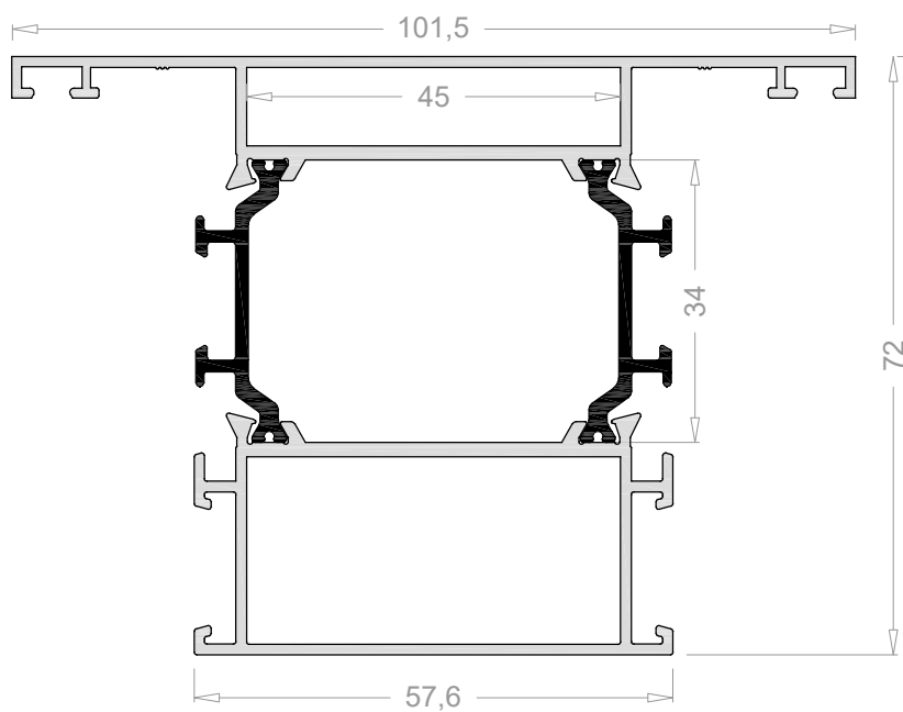
Travesaño de 102 mm 4308
