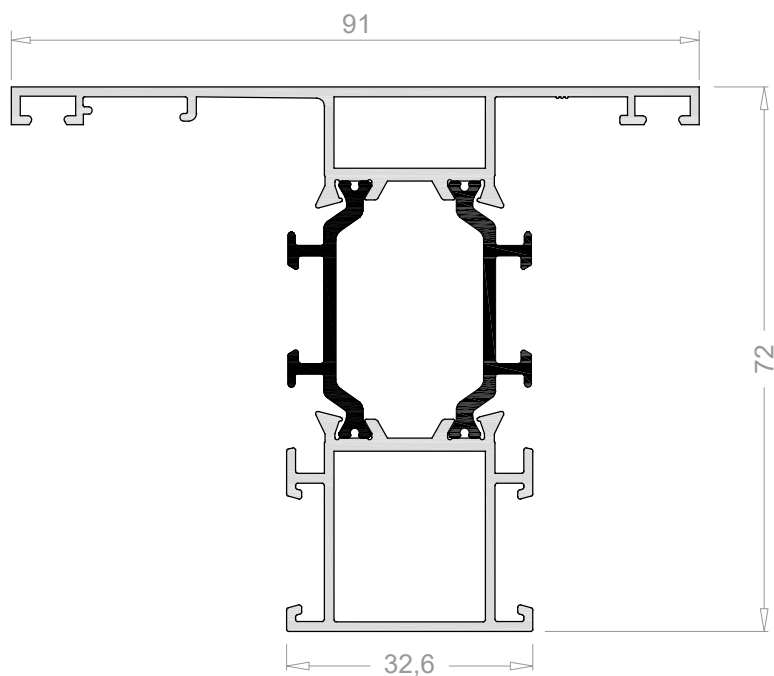
Travesaño asimétrico de 91 mm
