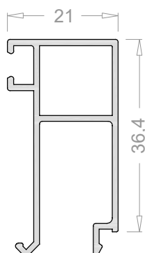
Junquillo recto alto de 21 mm 3311
