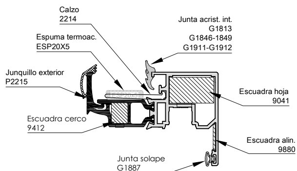
Hoja Recta 31 mm 3302
