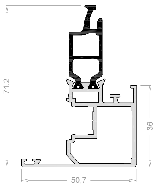
Hoja Recta 31 mm 3302
