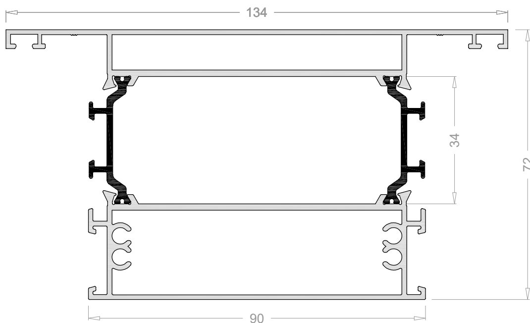
Travesaño ó zócalo de 134 mm
