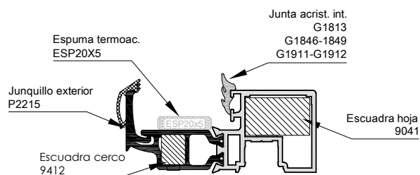
Hoja Inversora 35 mm 3305
