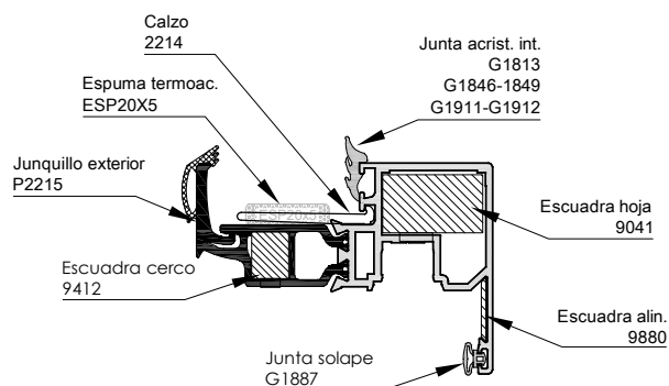
Hoja Recta 35 mm 3304
