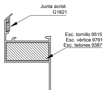
Cerco con solape ( 25 mm) 3575
