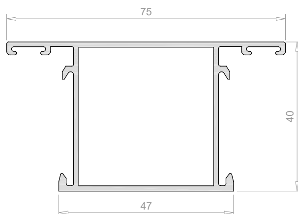
Travesaño de 75 mm
