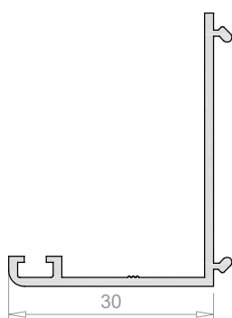
Solape de 30 mm
