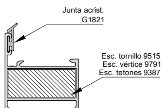
Cerco 3501
