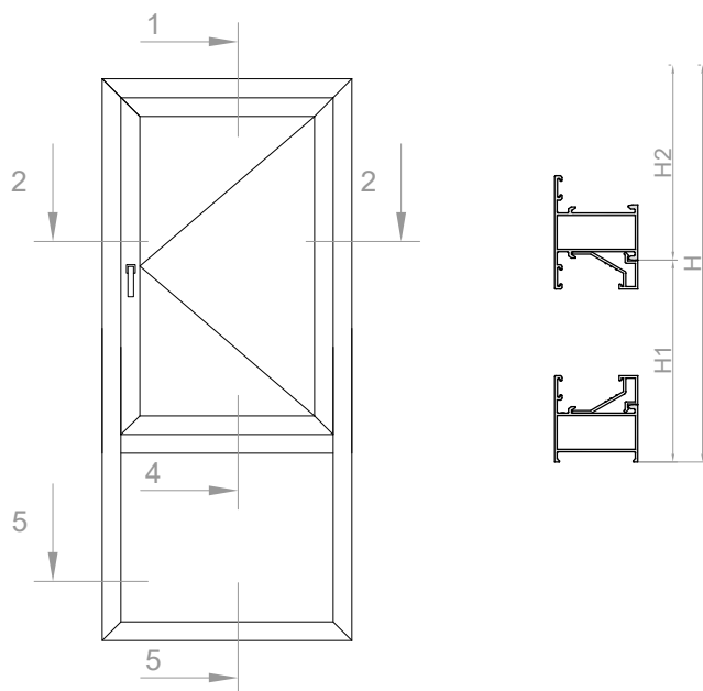
VENTANA - Una hoja + fijo
