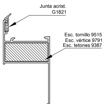
Cerco con solape ( 35 mm) 3531
