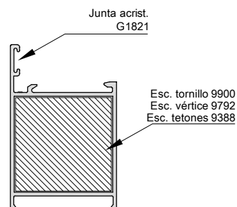
Cerco reforzado 3507
