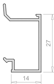
Junquillo de 27 mm 3560
