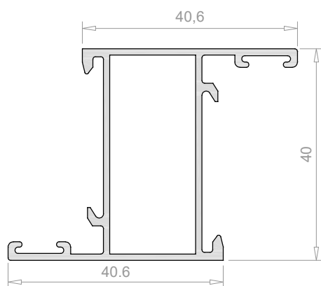
Hoja recta de ventana 3502
