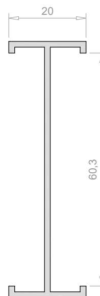
Unión de cercos de 60 mm
