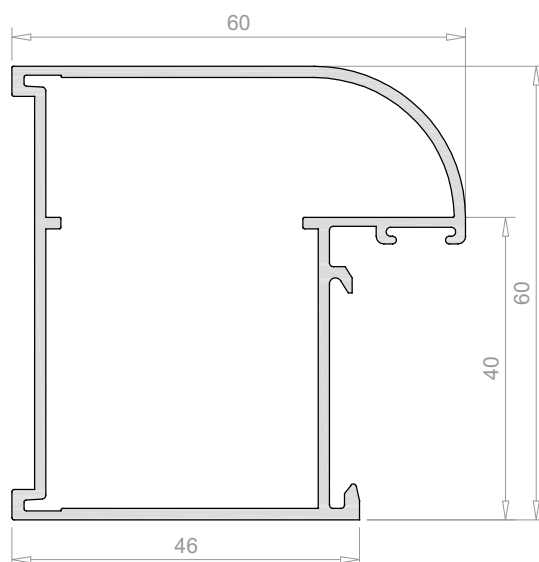
Cerco con forma 3583
