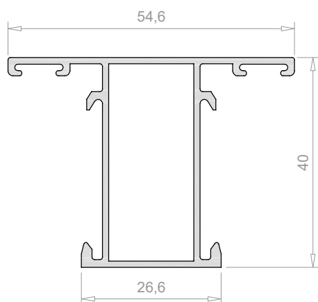
Inversor y travesaño de 55 mm
