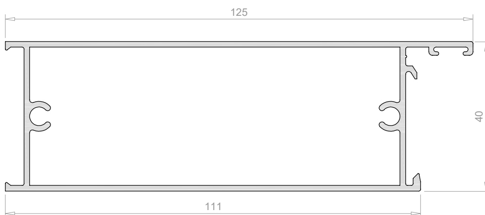
Zócalo puerta 3512
