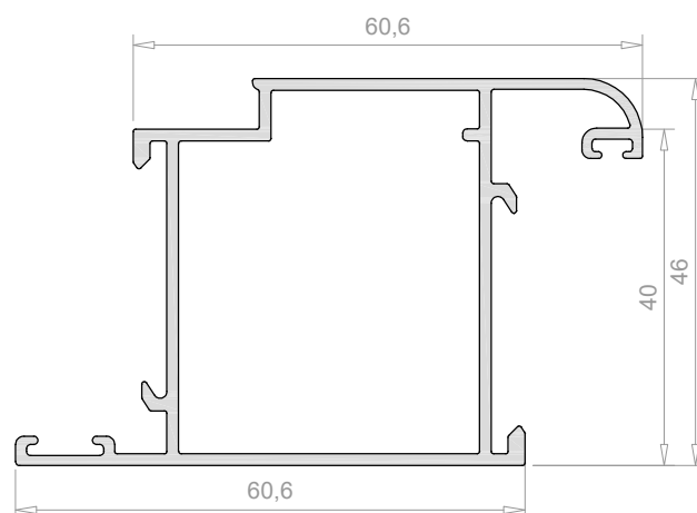
Hoja curva puerta 3585
