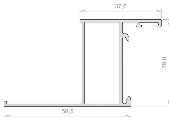
Cerco con solape(35 mm) 3531
