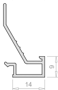
Junquillo de 9 mm 3563
