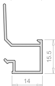
Junquillo de 15 mm 3562
