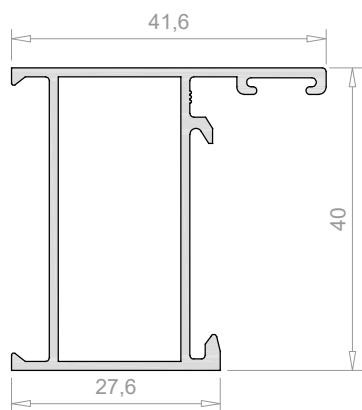
Cerco 3501
