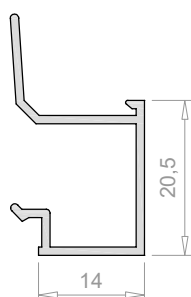
Junquillo de 20 mm 3566
