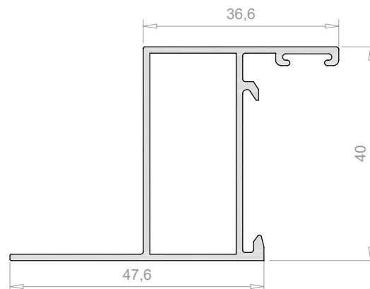
Cerco con solape(25 mm) 3575
