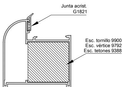
Cerco con forma 3583
