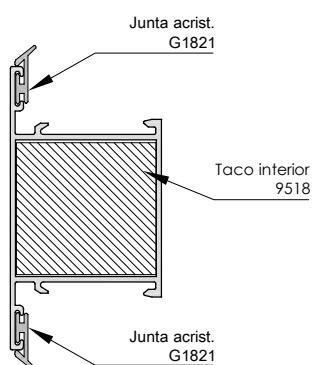
Travesaño de 75 mm 3511
