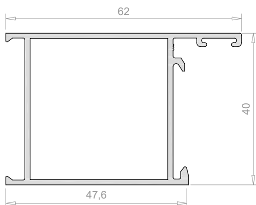
Cerco reforzado 3507
