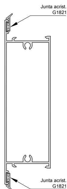
Travesaño de 55 mm 3513
