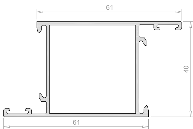
Hoja recta puerta 3508
