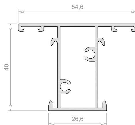
Travesaño de 55 mm con portatornillos
