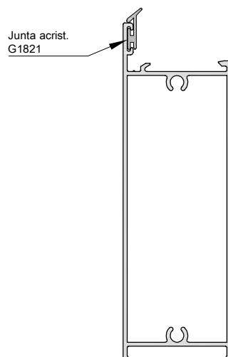
Zócalo de puerta 3512
