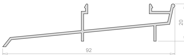
Perfil recogecondesaciones con vierteaguas
