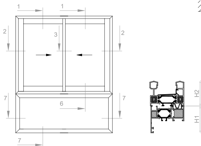
VENTANA - Dos hojas Hojas Corte Recto + Fijo
