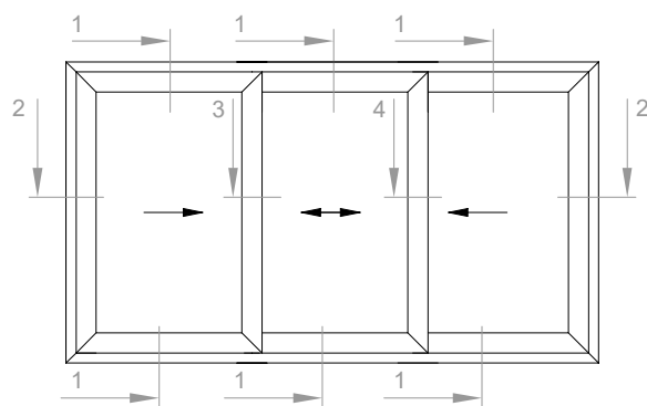
VENTANA - 3 hojas - Cerco tricarril Hojas Perimetrales
