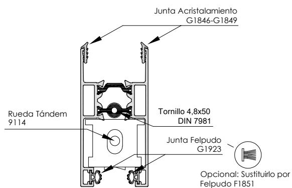
Hoja Horizontal 3612
