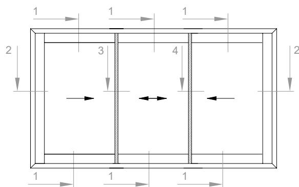
VENTANA - 3 hojas - Cerco tricarril Hojas Corte Recto - Cruce de 23 mm
