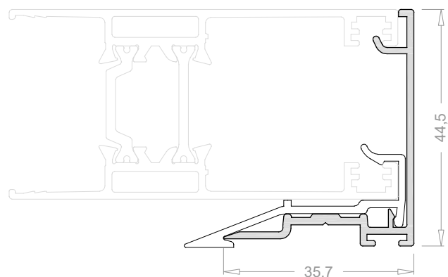
Enganche de hoja perimetral 3621
