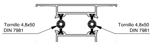
Parteluz Hoja 3616
