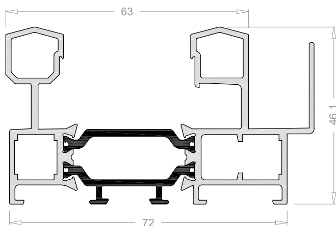
Cerco de 72 con recogecondesación 3605
