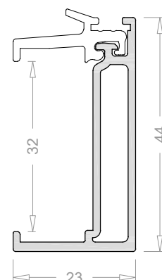
Hoja cruce 23 mm 3617
