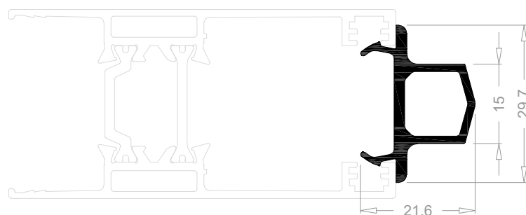
Unión de hojas enfrentadas PVC P3626
