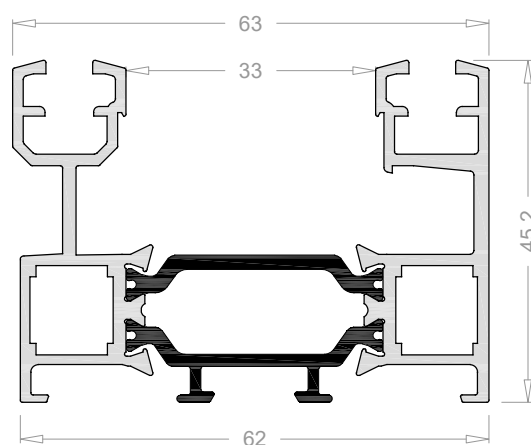
Cerco de 62 mm abierto 3602
