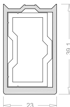
Refuerzo de hoja 23 mm 3628
