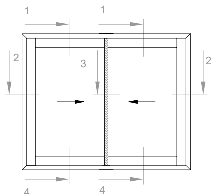
VENTANA - Dos hojas Hojas Corte Recto - Cruce 23 mm
