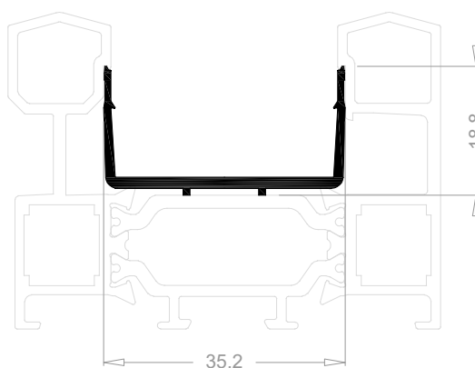
Perfil "U" PVC P3624
