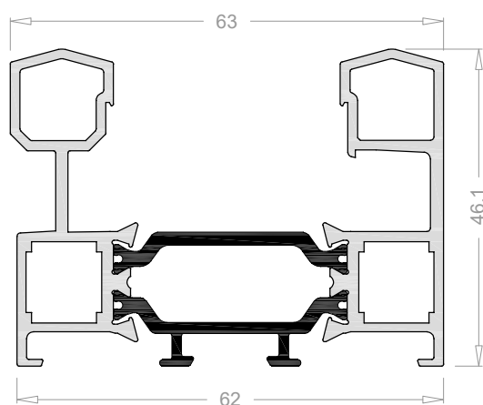
Cerco de 62 mm 3601
