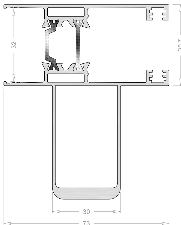
Hoja perimetral de cruce reforzada 3623
