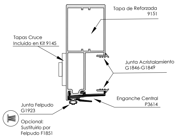
Hoja de Cruce Reforzada 3615
