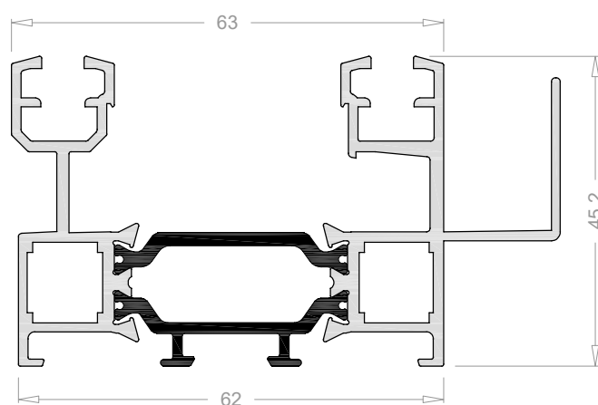
Cerco de 62 abierto con recoge. 3604
