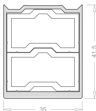
Refuerzo de hoja 3627
