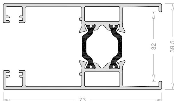
Hoja lateral 3611
