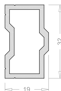
Refuerzo modular interior 3629
