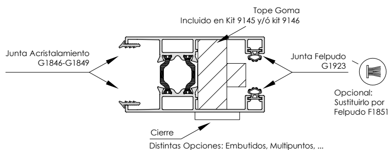
Enganche de PVC para 3621 P3622
