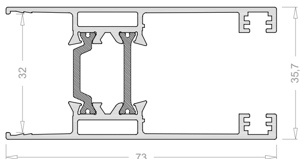
Hoja perimetral 3620
