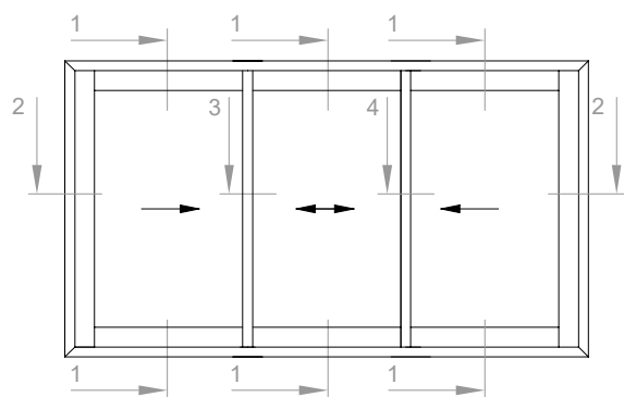
VENTANA - 3 hojas - Cerco tricarril Hojas Corte Recto
