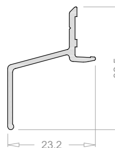
Vierteaguas 3610
