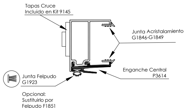
Hoja de Cruce 3613
