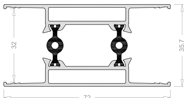
Partelunas 3616
