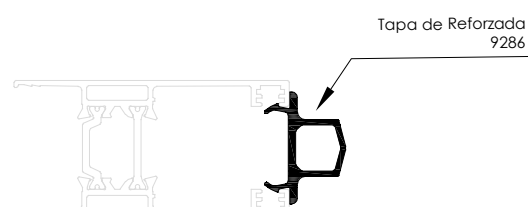
Unión de Hojas Enfrentadas PVC P3623
