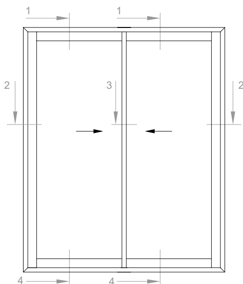
BALCONERA - Dos hojas Hojas Corte Recto
