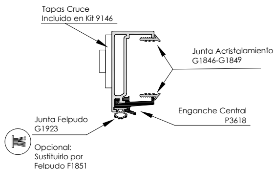
Hoja de Cruce de 23 mm 3617
