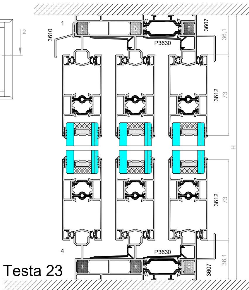
VENTANA - 3 hojas - Cerco tricarril Hojas Corte Recto - Cruce de 23 mm
