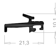
Enganche cruce 23 mm P3618
