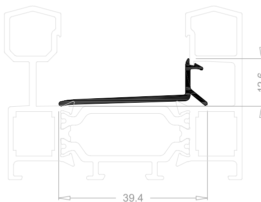
Perfil "L" PVC P3630
