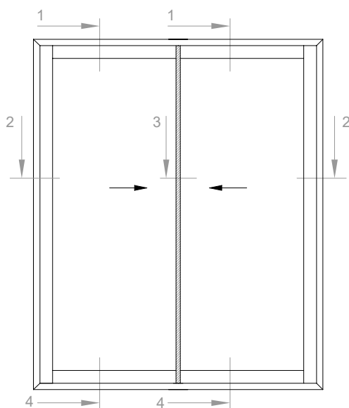
BALCONERA - Dos hojas Hojas Corte Recto - Cruce de 23 mm
