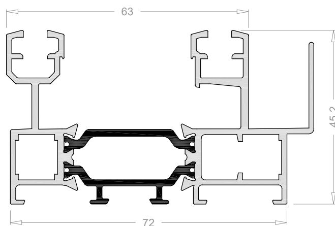
Cerco de 72 abierto con recoge. 3606
