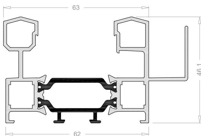
Cerco de 62 con recogecondesación 3603
