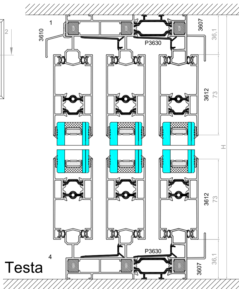
VENTANA - 3 hojas - Cerco tricarril Hojas Corte Recto
