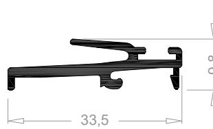
Enganche de cruce P3614
