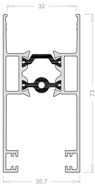
Hoja horizontal 3612
