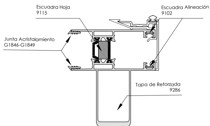
Hoja Perimetral de Cruce Reforzada 3623
