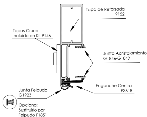
Hoja de Cruce Reforzada de 23 mm 3619
