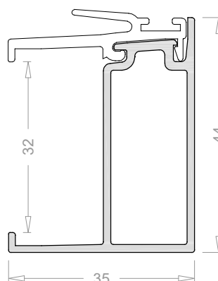
Hoja de cruce 3613
