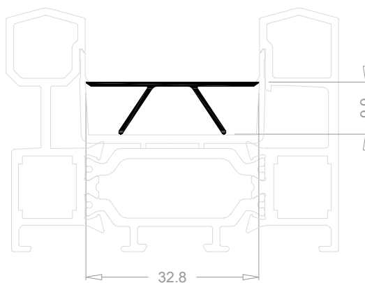
Perfil tapa de "U" PVC P3625
