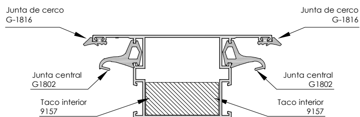
Travesaño intermedio ( para apertura en ambos lados ) 4586
