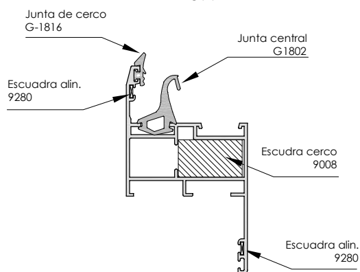
Cerco son solape ( 30 mm ) 4599
