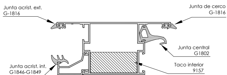
Travesaño intermedio ( para apertura y fijo ) 4586
