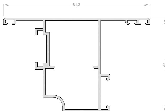
Hoja de apertura exterior 4598
