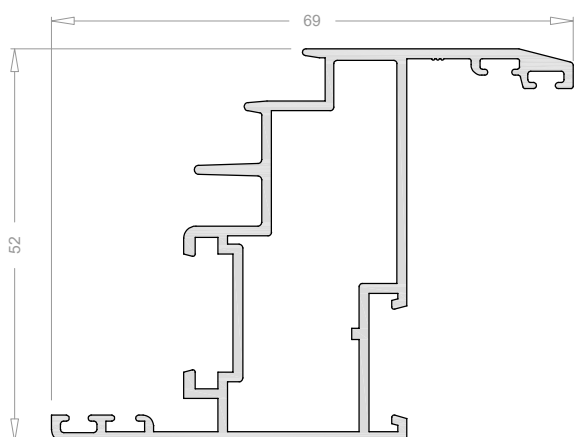
Hoja de ventana 4582
