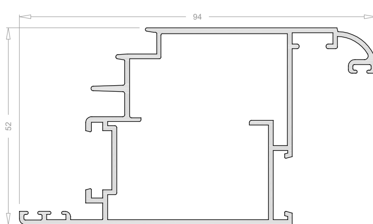
Hoja curva puerta 4601
