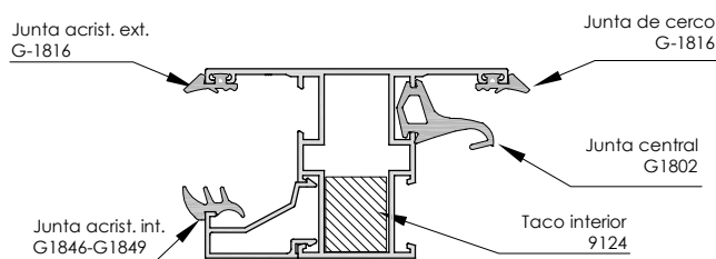
Travesaño estrecho ( para apertura y fijo ) 4585
