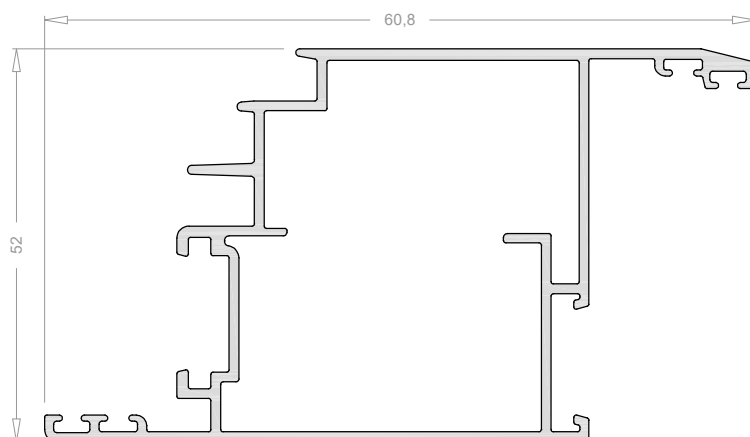
Hoja recta puerta 4584
