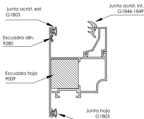
Hoja Apertura Exterior 4598
