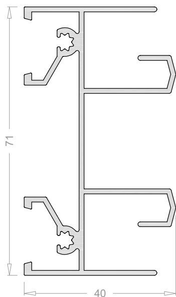
Cerco superior a testa 5001
