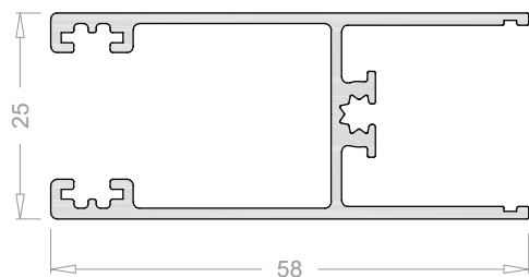
Hoja horizontal 22 mm 5006
