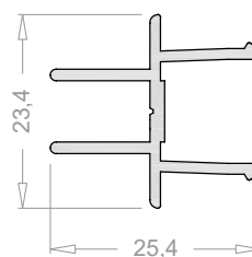
Acople hojas enfrentadas 5017
