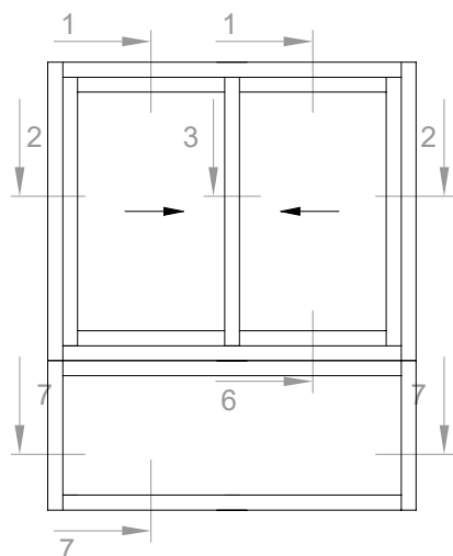
VENTANA - Dos hojas + fijo
