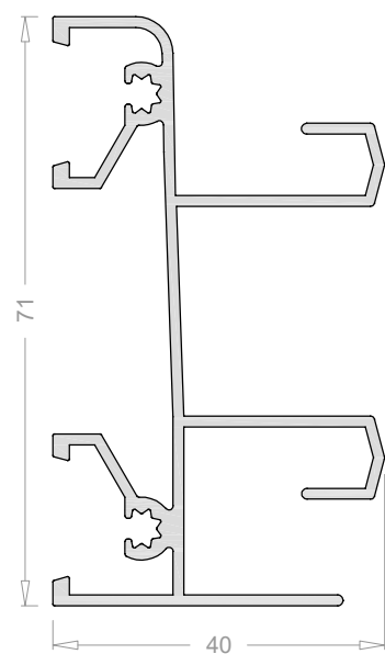
Cerco inferior a testa 5003
