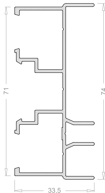
Cerco lateral a testa 5002
