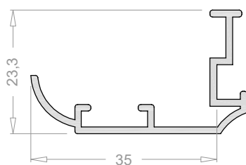
Solape con forma de 35 mm 5026
