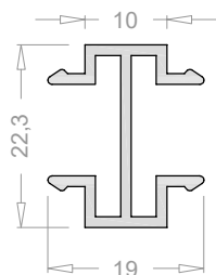
Perfil unión cercos clipado 5031
