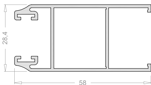
Hoja lateral 22 mm 5005
