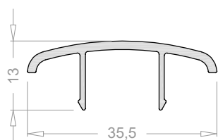
Tapa de refuerzo 6842
