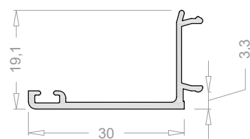
Solape de 30 mm 2519
