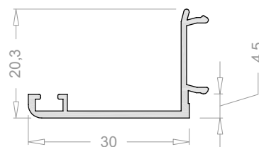
Solape de 30 mm 2518
