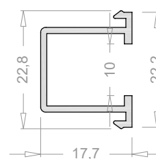
Reductor vidrio (de 22 a 10 mm) 5019
