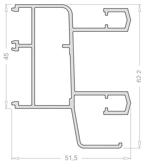
Cerco perimetral de 45 mm 5020
