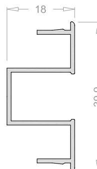
Reductor 5103
