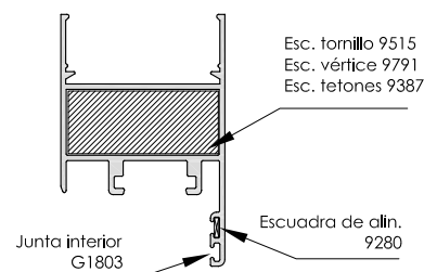
Lama 5104
