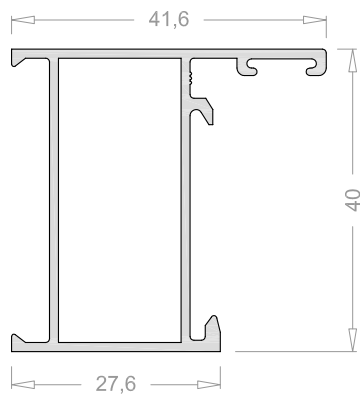
Cerco 3501
