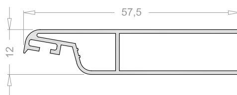
Compensador 5105
