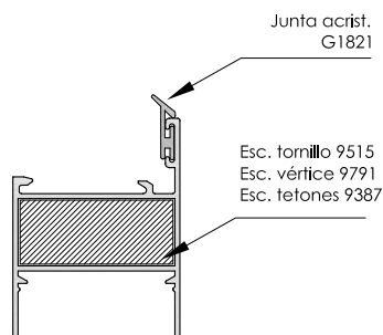
Cerco - Hoja 5101
