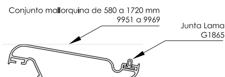
Lama 5104
