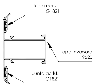
Inversor 3506
