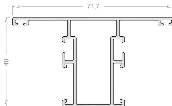
Travesaño para fijo cámara europea 2516
