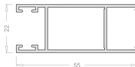
Hoja lateral 17 mm 6539
