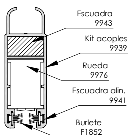
Hoja perimetral 10 mm 6560
