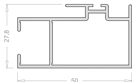
Hoja central 10 mm 6531
