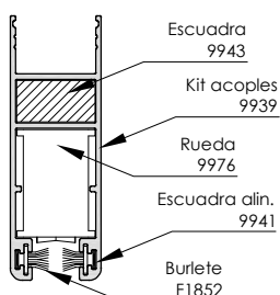
Hoja perimetral 19 mm 6561
