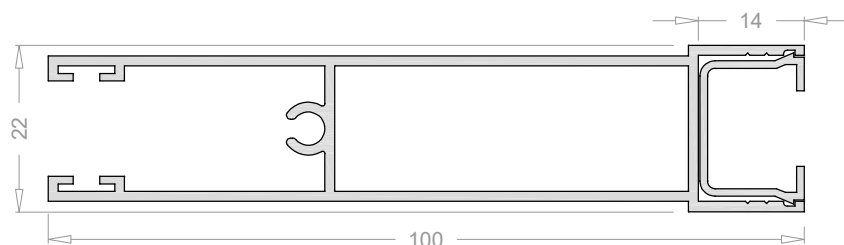
Hoja horizontal reforzada 19 mm 6511
