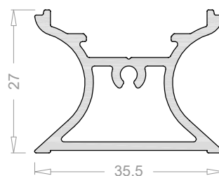
Refuerzo para cruce 6843
