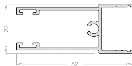
Hoja horizontal 19 mm 6507
