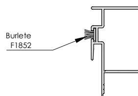
Hoja central 19 mm 6508
