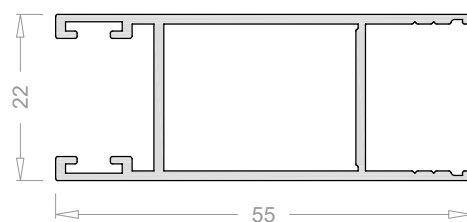
Hoja lateral 19 mm 6509
