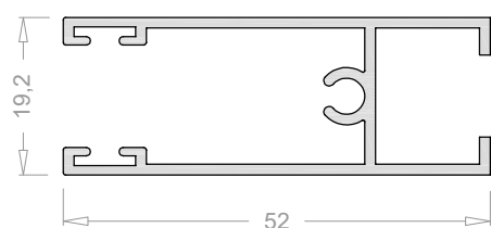
Hoja horizontal 10 mm 6530
