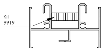
Cerco superior (testa) 6541
