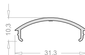
Tapa curva para cerco lateral 6554
