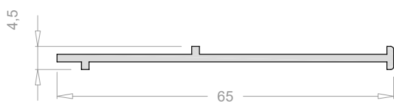
Perfil unión cercos (6500+3500) 6515
