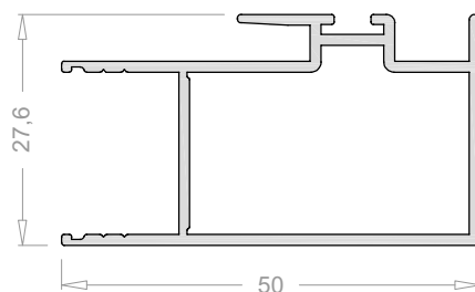
Hoja central 19 mm 6508
