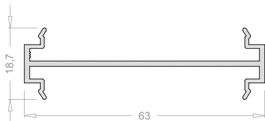
Perfil de unión de cercos (6500) 6547
