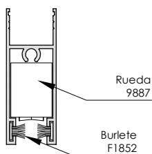
Hoja horizontal 17 mm 6537
