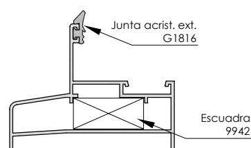
Cerco para fijo perimetral 6569
