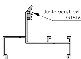
Cerco para fijo 6525
