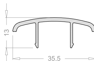
Tapa de refuerzo 6842
