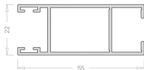
Hoja lateral 10 mm 6532
