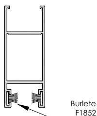
Hoja lateral 17 mm 6539
