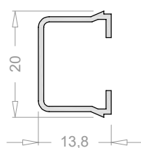
Reductor vidrio (de 19 a 10 mm) 6514
