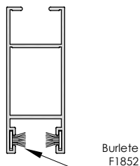
Hoja lateral 10 mm 6532
