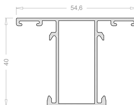
Travesaño para fijo (5361) 3506
