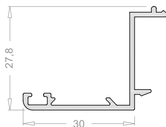
Solape de 30 mm 6521
