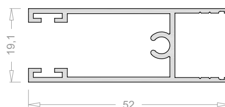
Hoja horizontal 17 mm 6537
