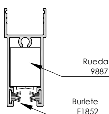
Hoja horizontal 19 mm 6507
