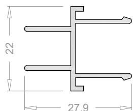
Acople hojas enfrentadas 6516
