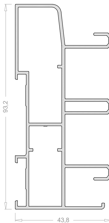
Cerco perimetral 3 carriles 6590
