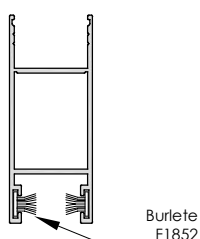
Hoja lateral 19 mm 6509
