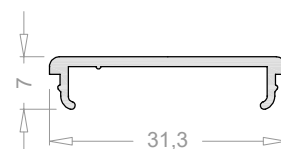
Tapa para cerco lateral 6518
