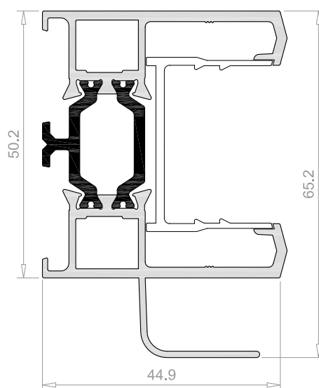
Cerco inferior perimetral de 50 con recogecondensaciones
