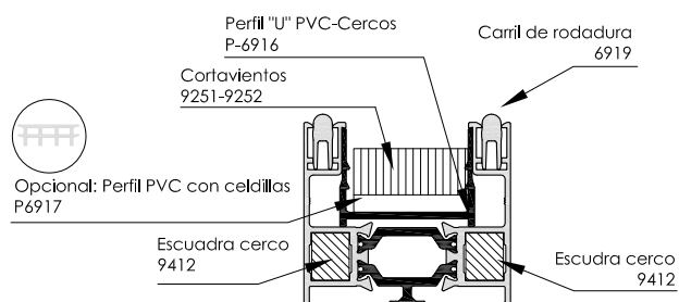
Cerco Perimetral de 50 mm 6920
