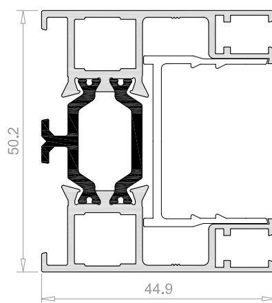
Cerco perimetral de 50 6914
