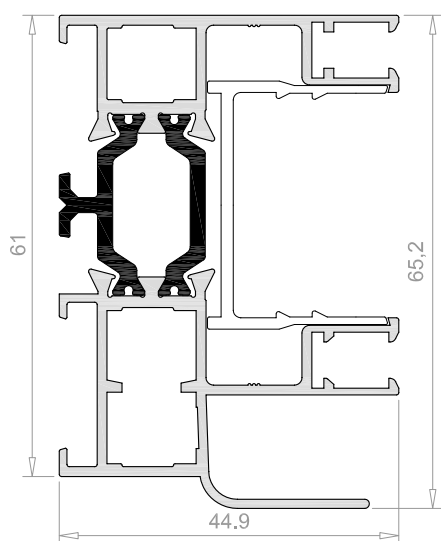
Cerco perimetral de 61 6920
