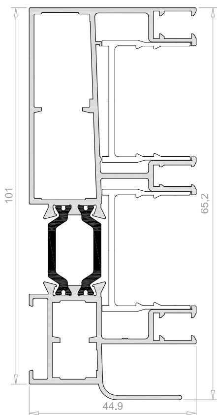
Cerco perimetral tricarril de 101 6921
