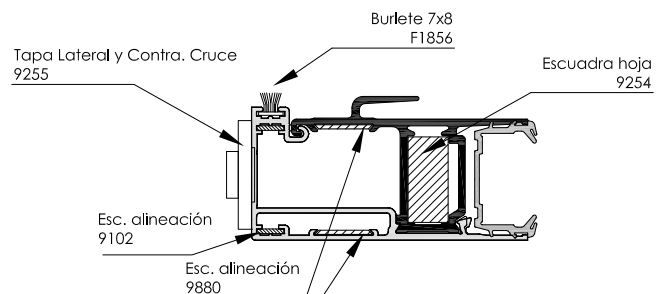
Hoja de cruce 6923
