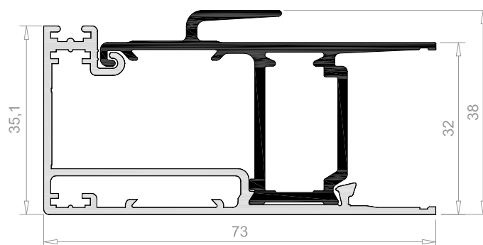
Hoja de cruce 6923
