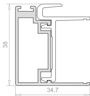
Hoja cruce interior 6911
