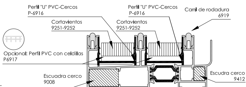
Cerco Perimetral tres carriles 6921
