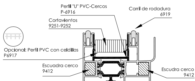
Cerco Perimetral de 61 mm 6920
