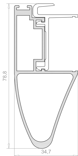
Hoja cruce interior reforzada 6907
