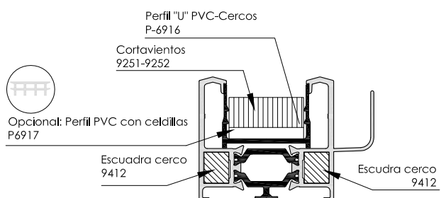
Cerco Perimetral 50 con condensación 6913
