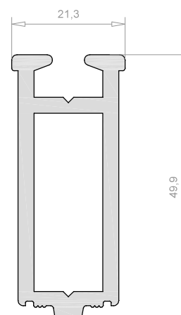
Perfil Acople 7607
