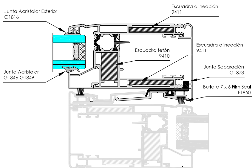
Hoja Perimetral + Cruce 7604 + 7605
