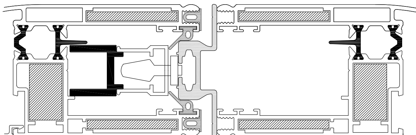
Detalle Encuentro 4 hojas
