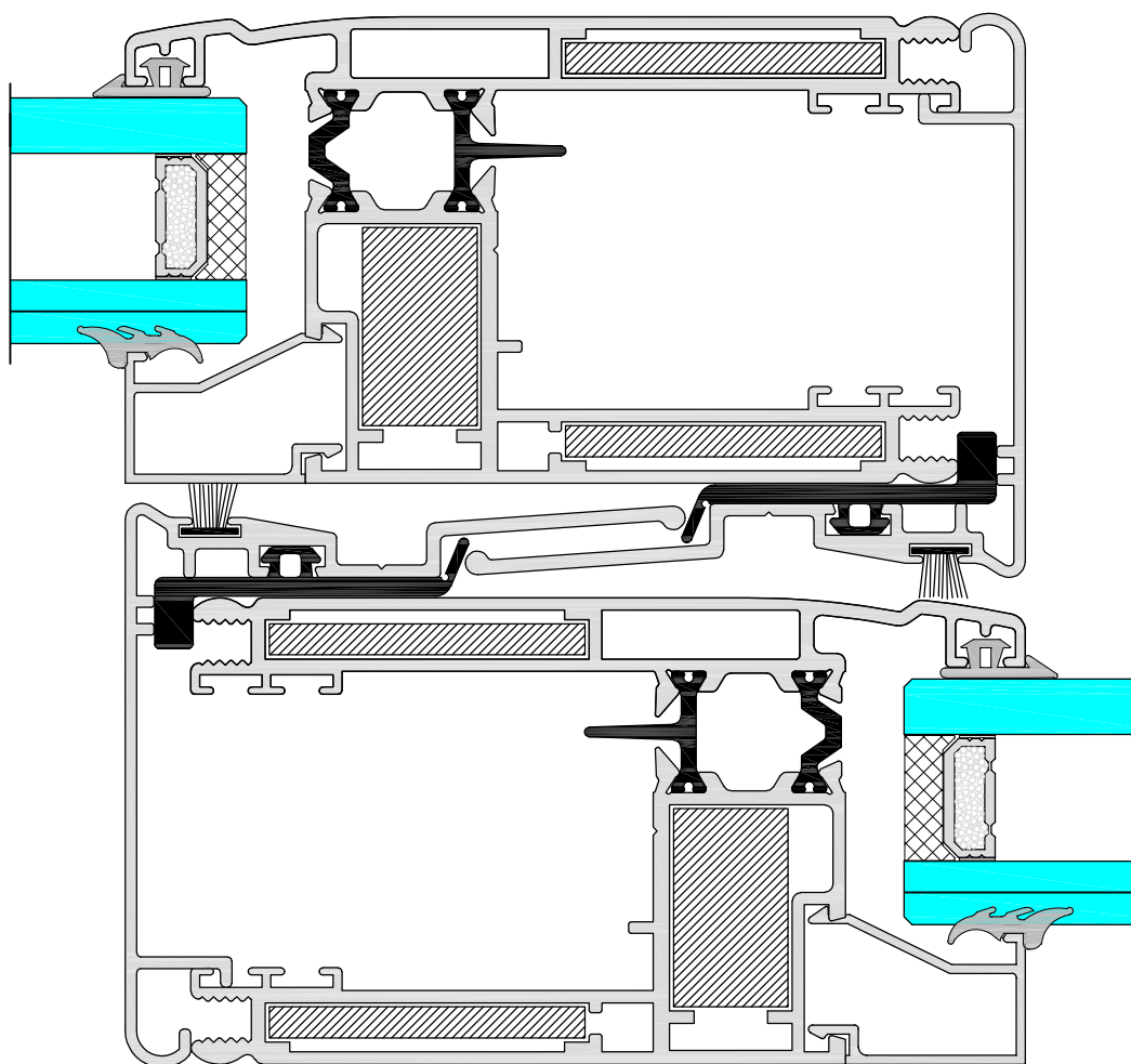
Detalle Nudo Central
