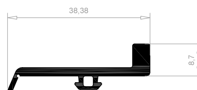
Perfil PVC Cruce G-1873
