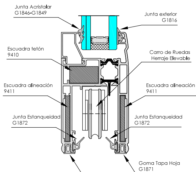
Hoja Perimetral 7604
