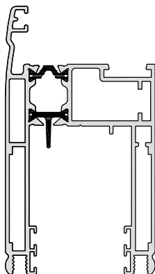
Hoja Perimetral 7604
