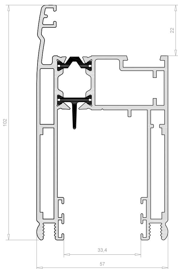
Hoja Perimetral 7604
