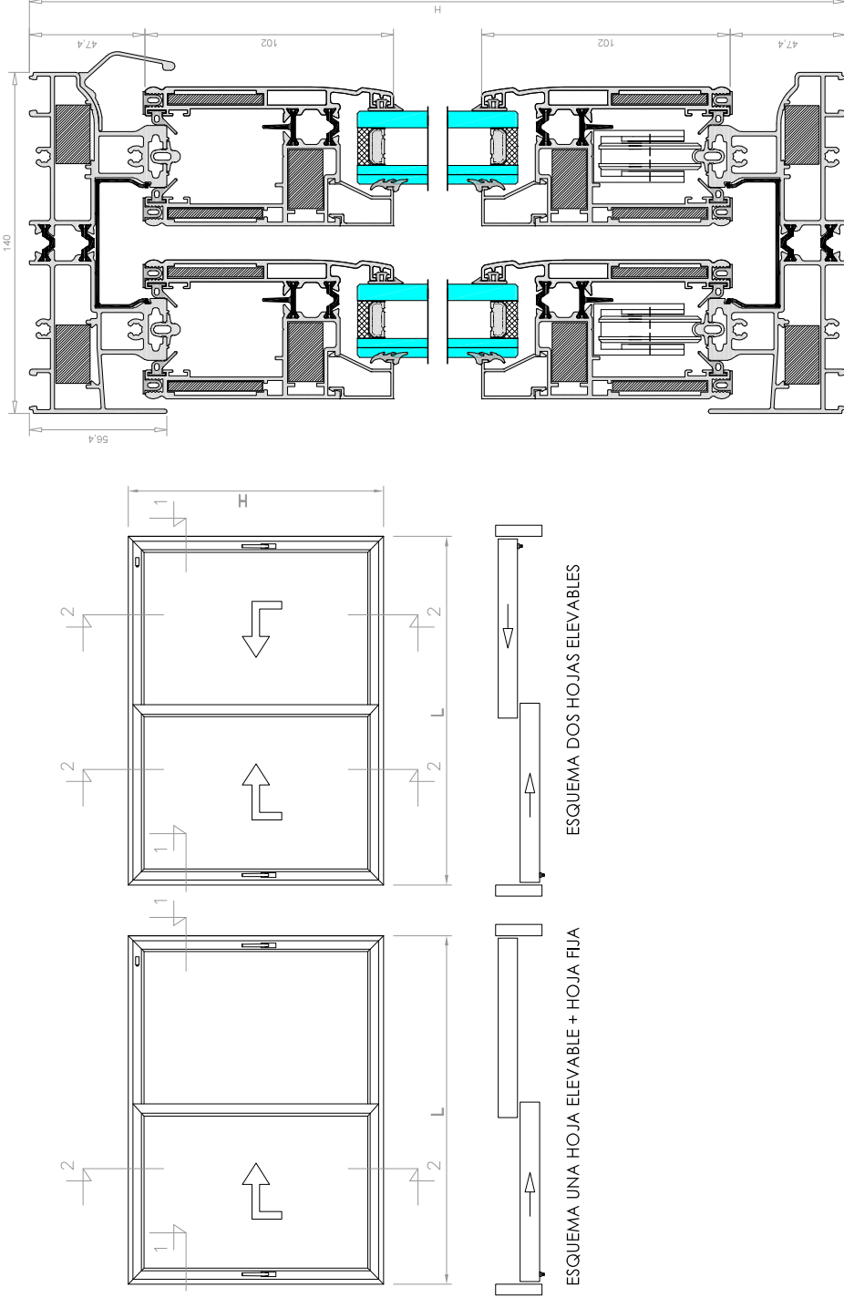
PERFILES CORREDERA ELEVABLE CE.43 P RPT Serie 7600
