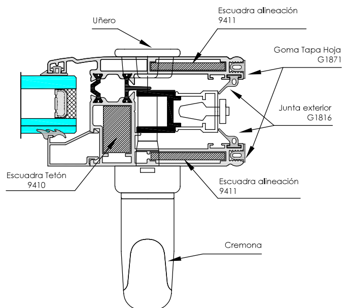
Hoja Perimetral Lateral 7604
