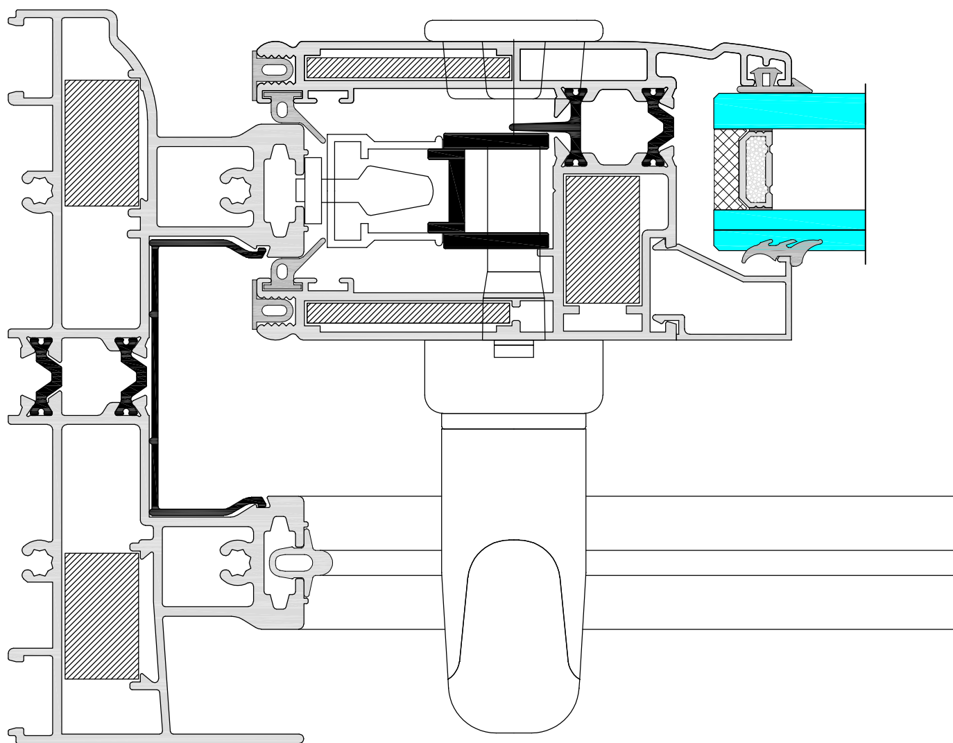
Detalle Nudo Lateral
