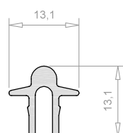
Carril de Rodadura 7609
